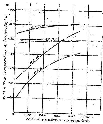
FIG. 1 Relação entre o nitreto de alumínio precipitado e os Tr15 e Tr5 do aço com 2,5% de Níquel
